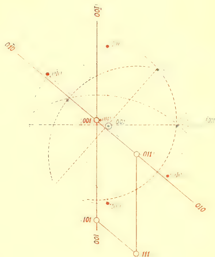
12. Клинопироксенъ.
